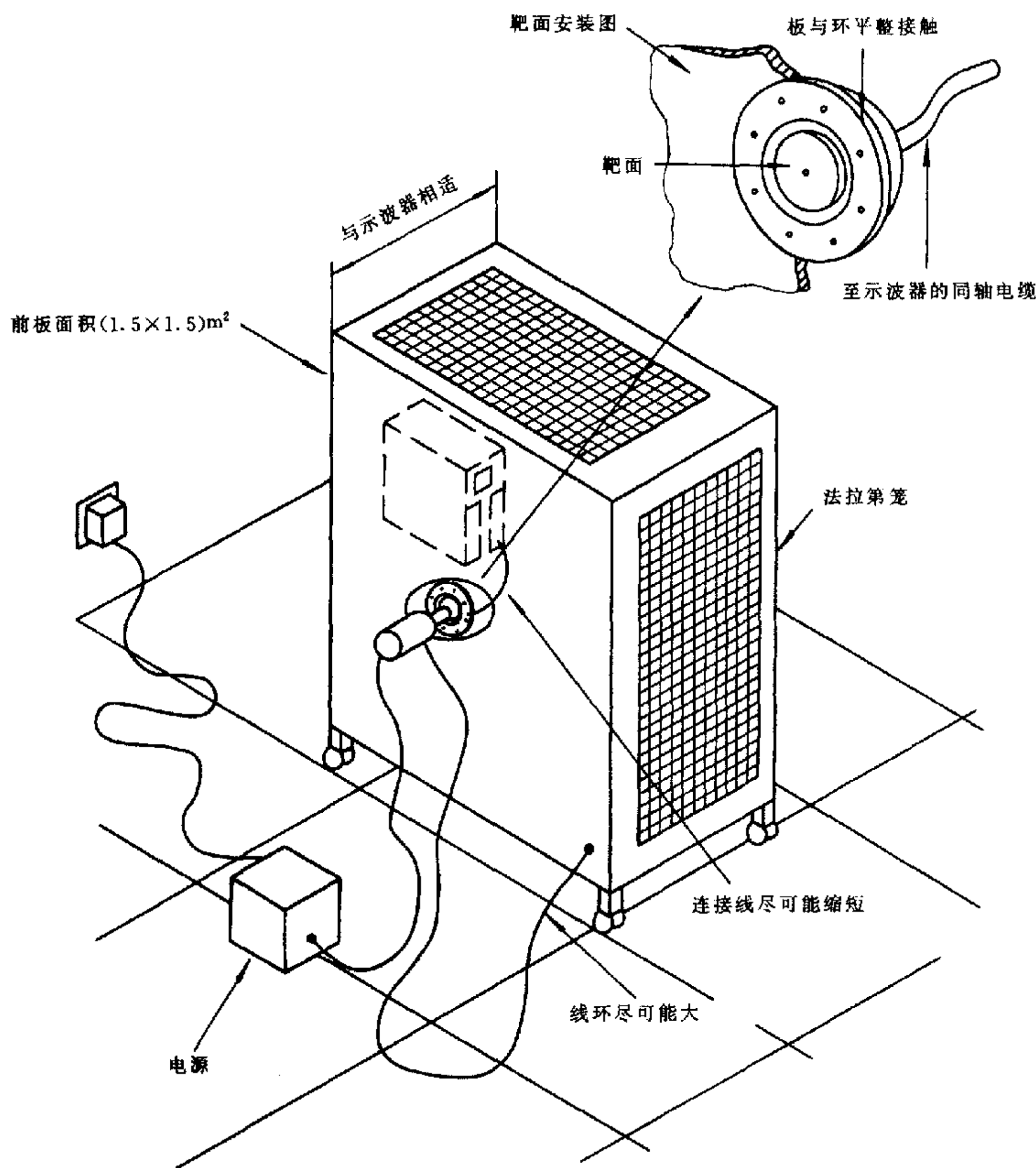
图 1 静电放电发生器简图
