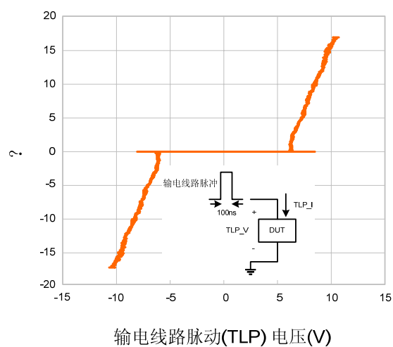
输电路脉动(TLP) 测量
