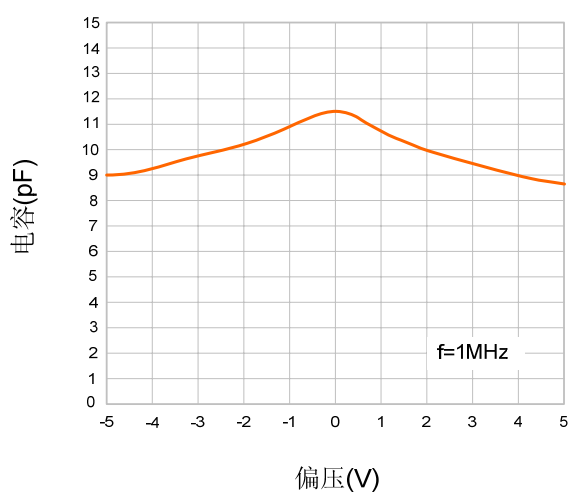
典型变化曲线 C_{IN} vs. V_{IN}
