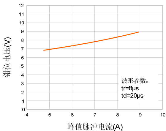
钳位电压 vs. 峰值脉冲电流
