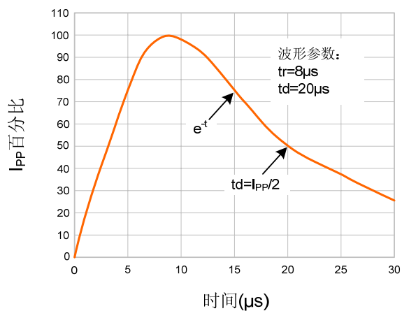
脉冲波形
