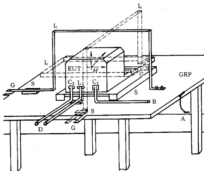
图3 台式设备的试验布置
