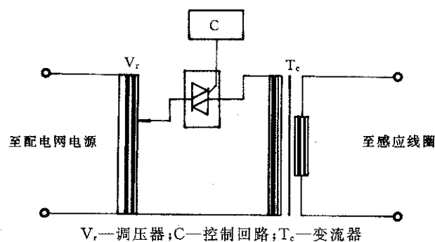
图2 工频磁场试验发生器的原理图
