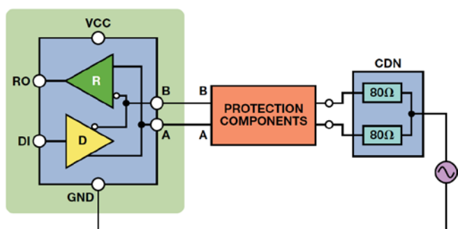
图 4. 半双工 RS-485 器件的耦合/去耦网络
