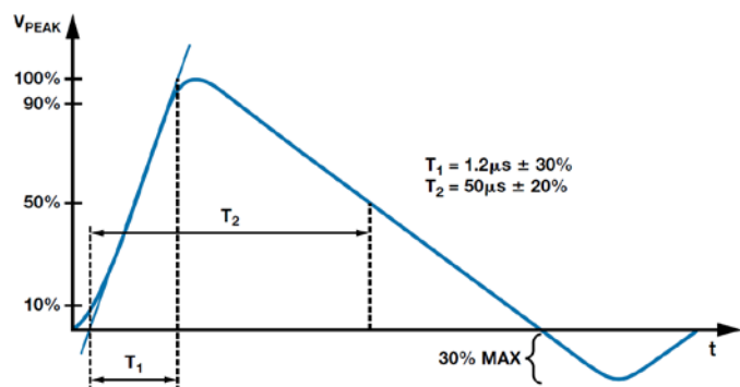
图 3. IEC 61000-4-5 电涌 1.2/50 \mu\text{s} 波形
