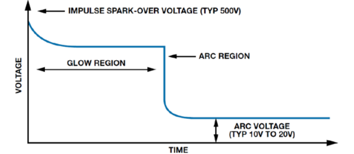
图 9. GDT 特性波形
