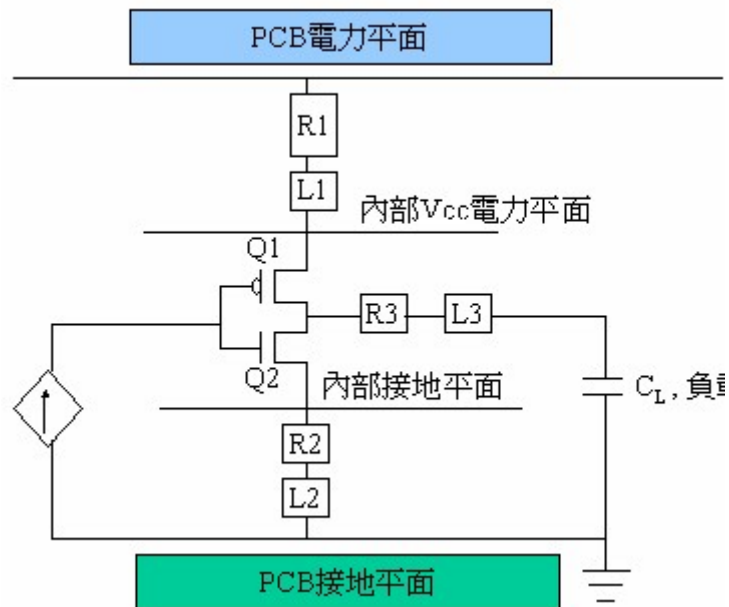
圖四：CMOS和PCB
