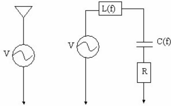
圖一：天線的等效電路
