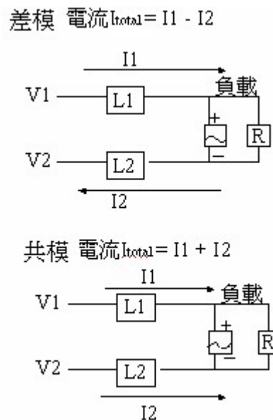
圖二：差模電流和共模電流
