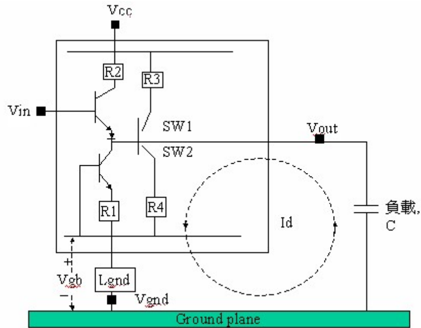
圖三：晶片內部的四個接腳和接地彈跳電壓
