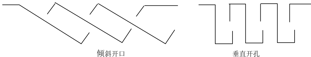
图 4B 防止垂直进入的开孔截面结构设计实例
