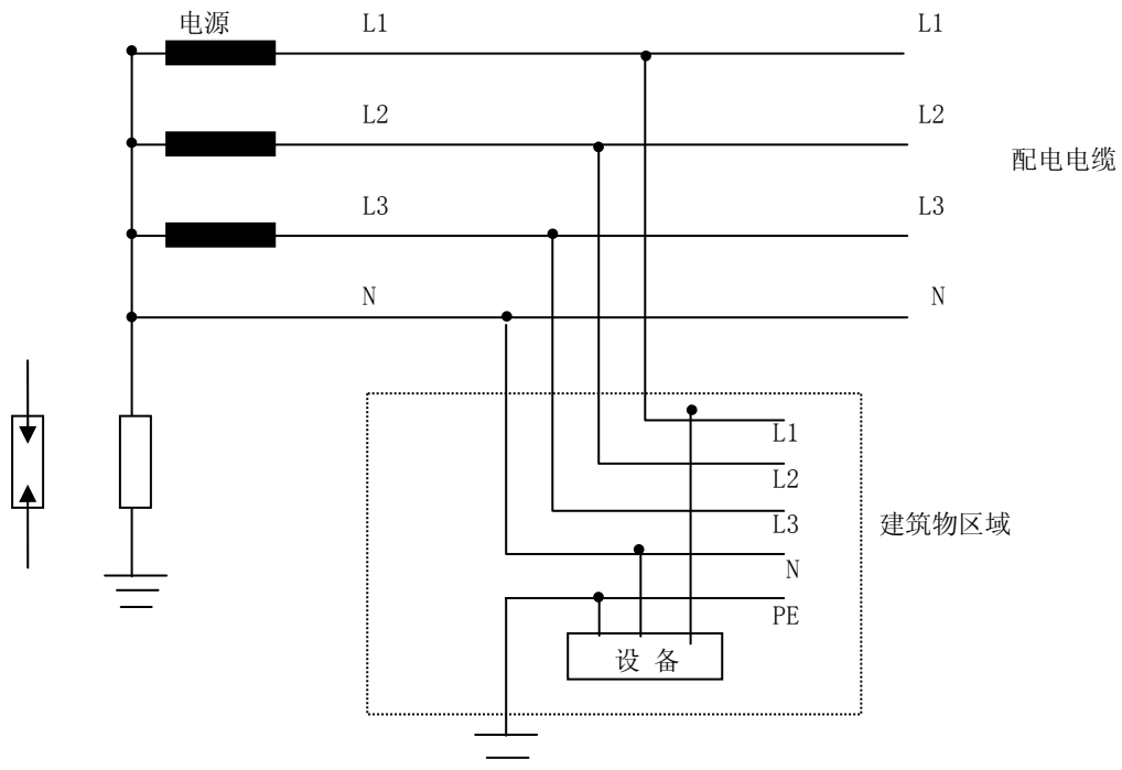
图 V7 三相线加中线的 IT 配电系统
