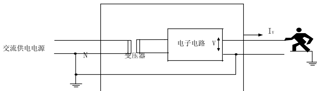
图 W2 接地电路的接触电流
