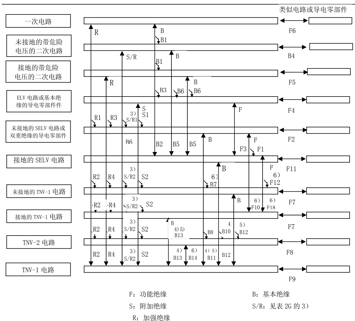
图 2F 绝缘应用实例
