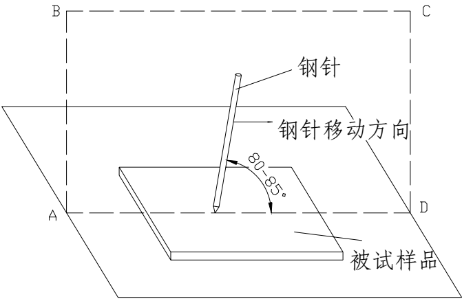
图 2H 涂层耐划痕试验
