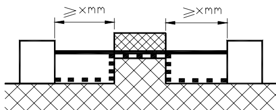
图 F5 带窄沟槽的未粘合接缝
