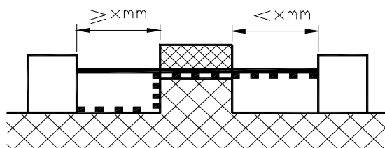
图 F6 带宽沟槽的未粘合接缝
