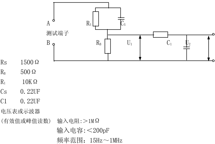
图 D1 测量仪器
