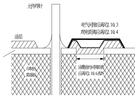
图 F11 印制线路板上的涂层
