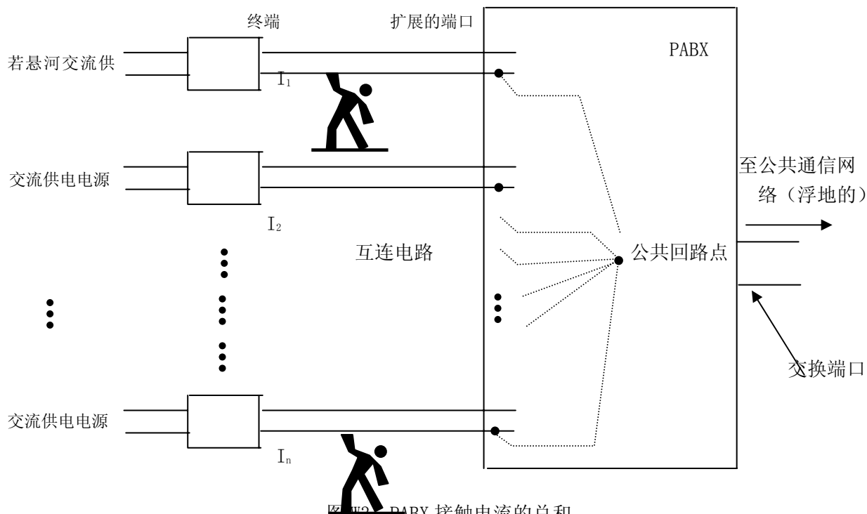
图 W3 PABX 接触电流的总和
