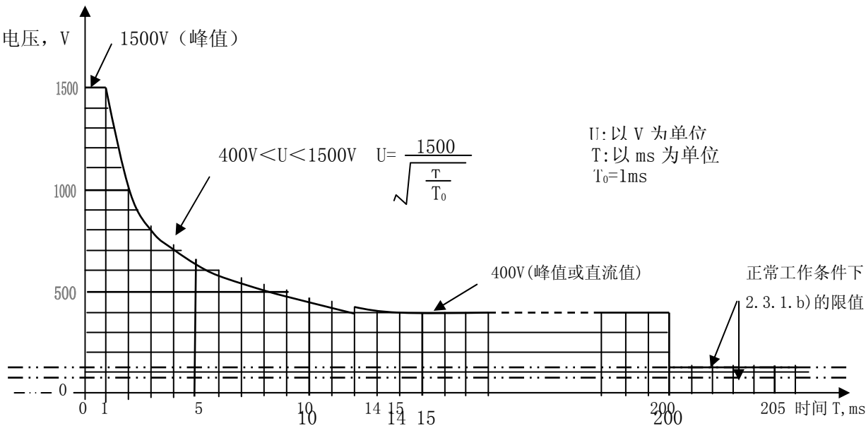
图示 D 单一故障后允许的最高电压
