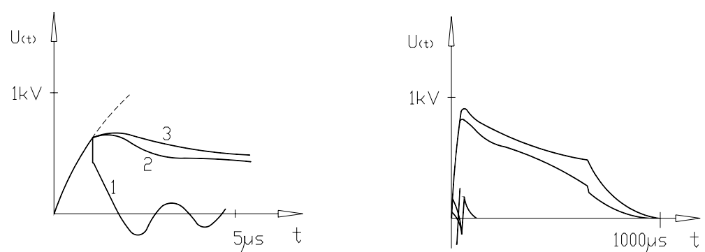
图 S2 不带电涌抑制器绝缘击穿时的波形
