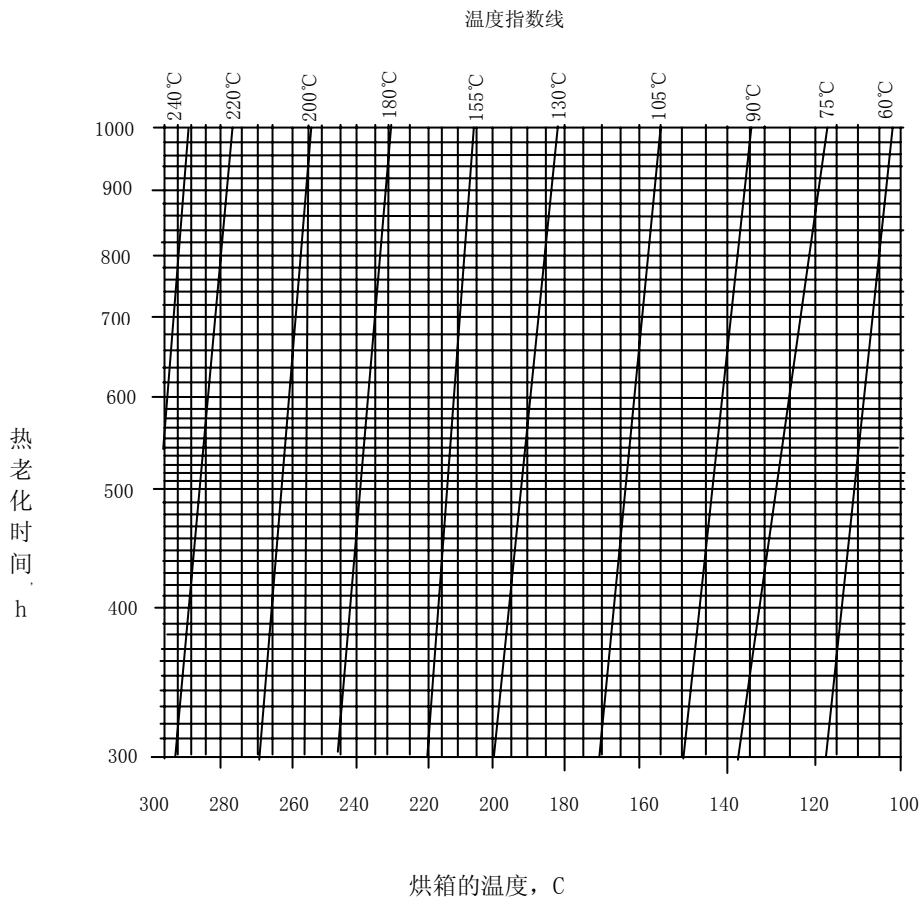
图 2G 热老化时间
