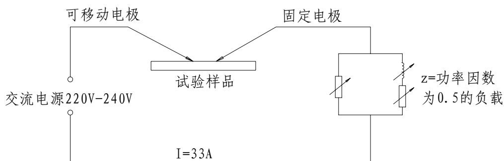
图 A1 大电流起弧试验电路
