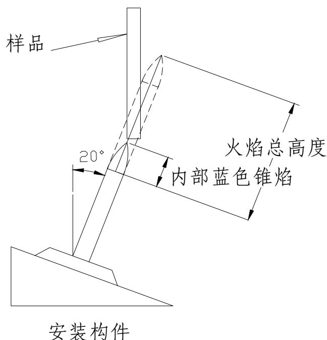
图 A4 5V 级材料的垂直燃烧试验示意图
