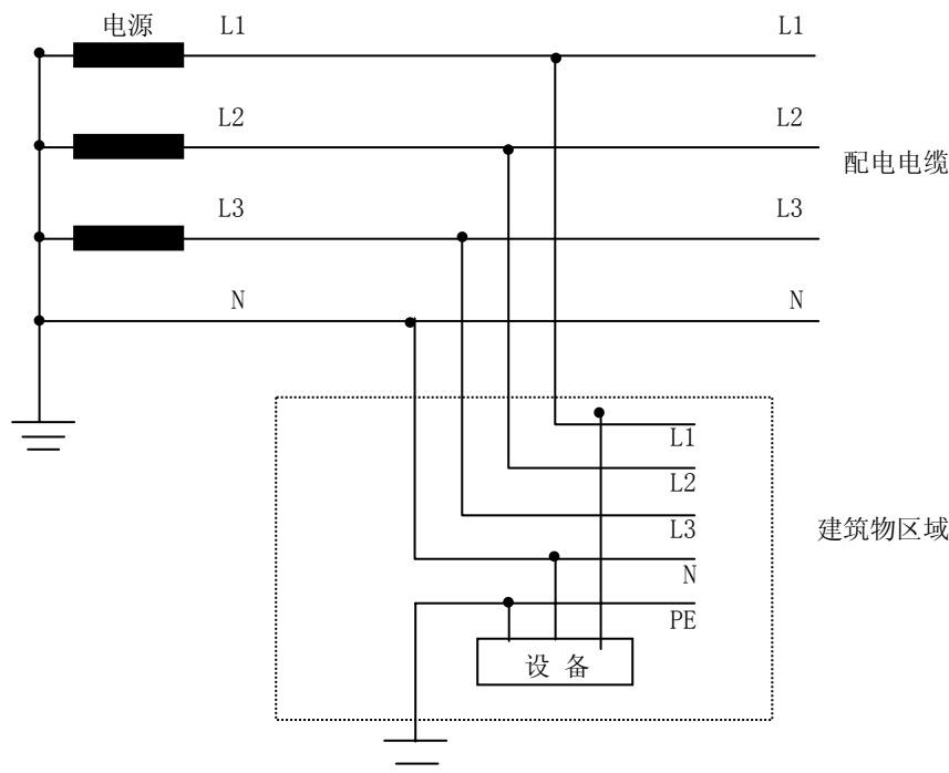
图 V5 三相线加中线的 TT 配电系统实例
