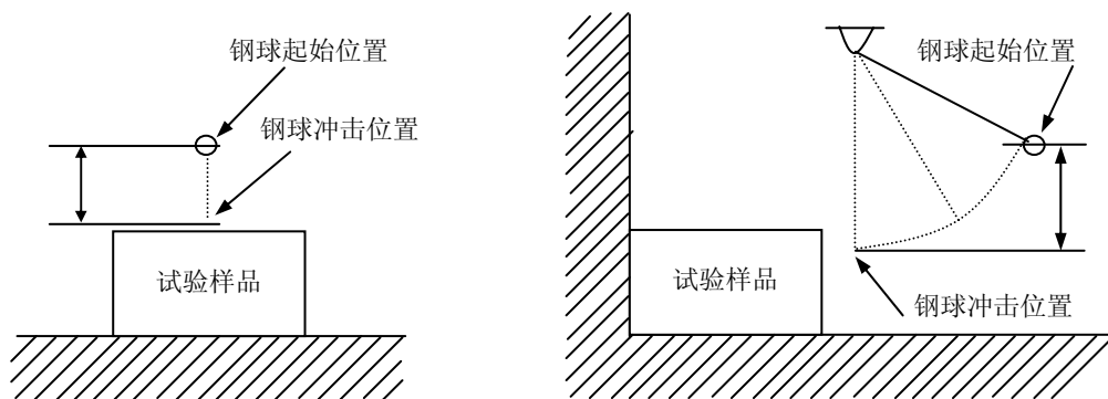
图 4A 钢球冲击试验
