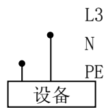
单独的中线和保护接地线 图 V1 TN-S 配电系统实例
