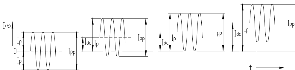
图 M3 峰值和峰-峰值电流
