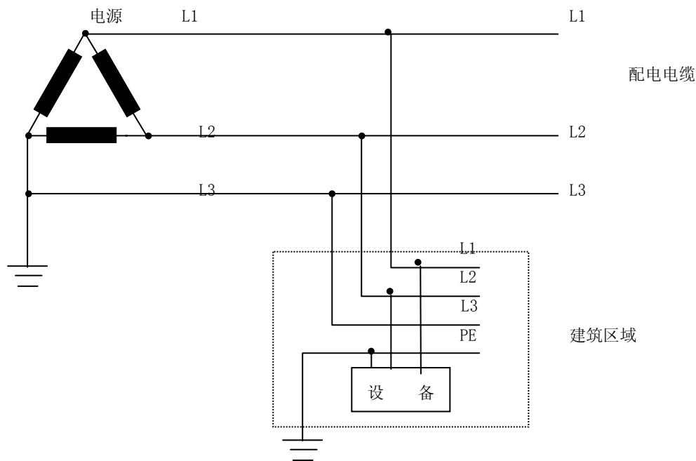
图 V6 三相线的 TT 配电系统
