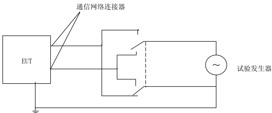
图 2E 试验电压发生器
