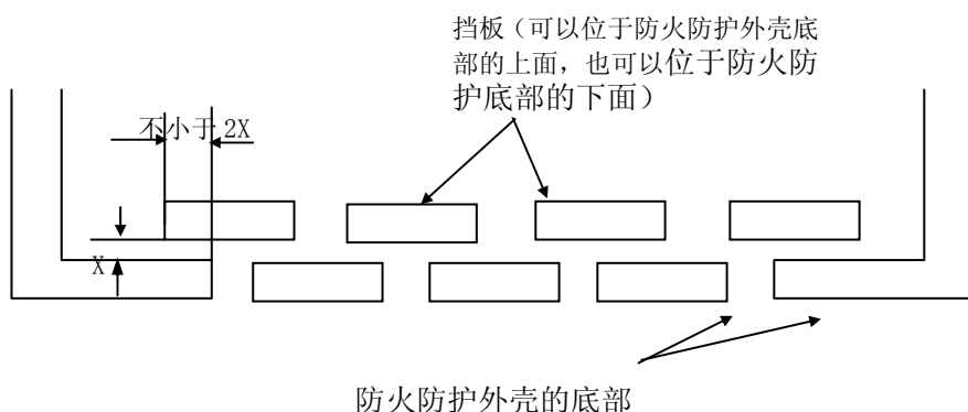
图表 F 挡板结构
