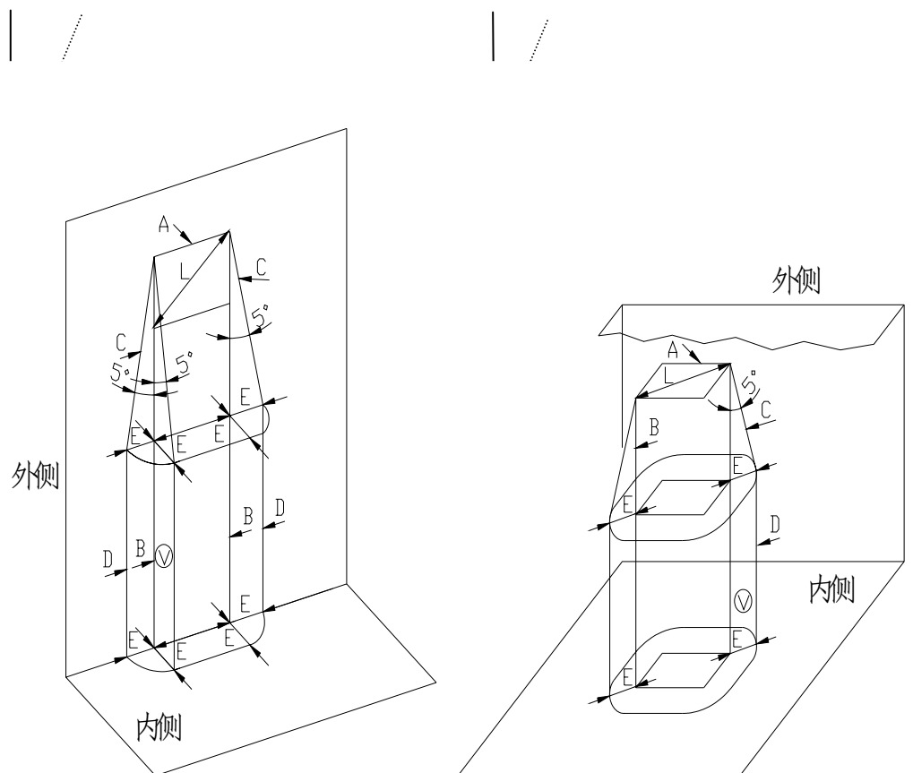
图 4B 防止垂直进入的开孔截面结构设计实例
