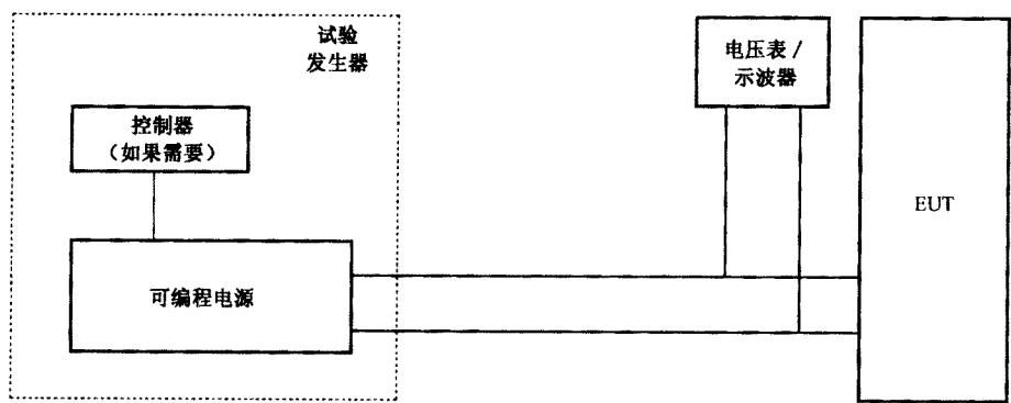
图 A. 2 以可编程装置为基础的发生器示例
