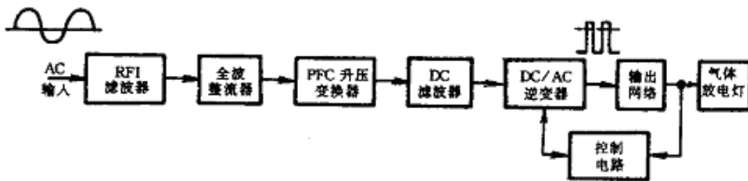
图 5 电子镇流器完整的电器原理方框图
