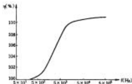
图 6 荧灯光效随频率变化曲线图
