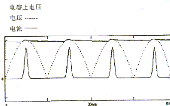
图 7 电容器电压、整流电压、电流波形
