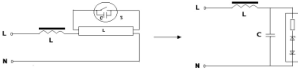
图 4 荧光灯稳态时的等效电路
