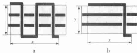
图 5 消除传输线干扰的方法
