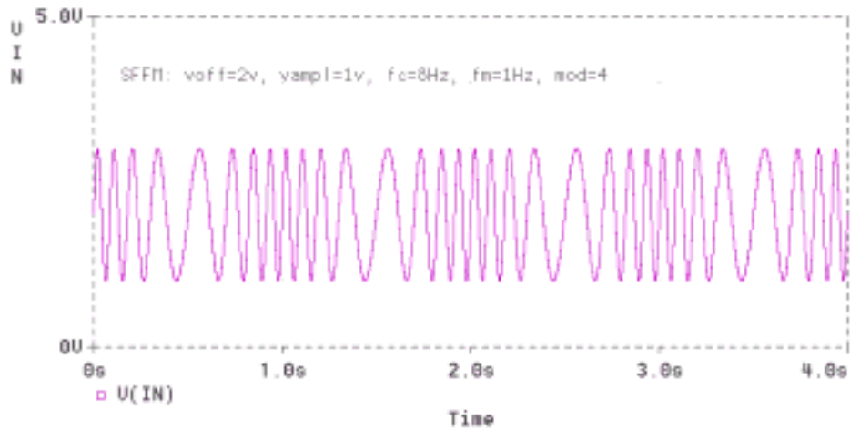
调频信号（例）
