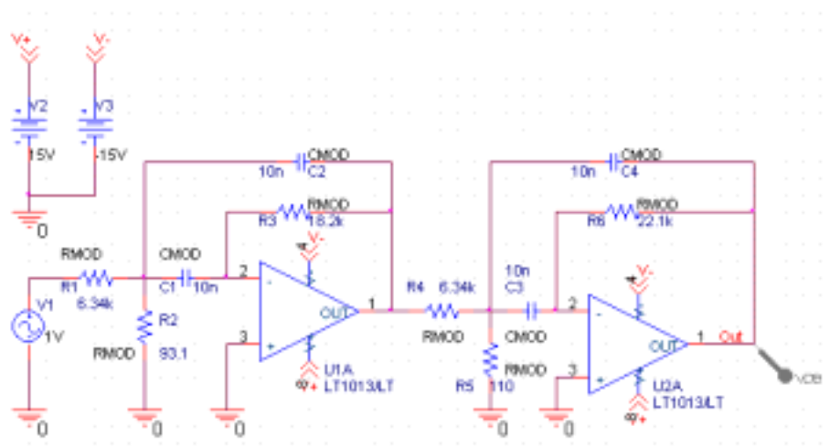
Chebyshev 有源滤波器
