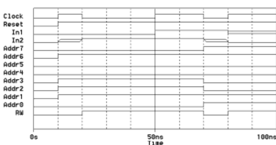
波形描述文件确定的信号波形(例 3)
