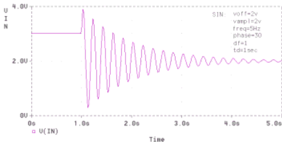
调幅正弦信号波形(例)
