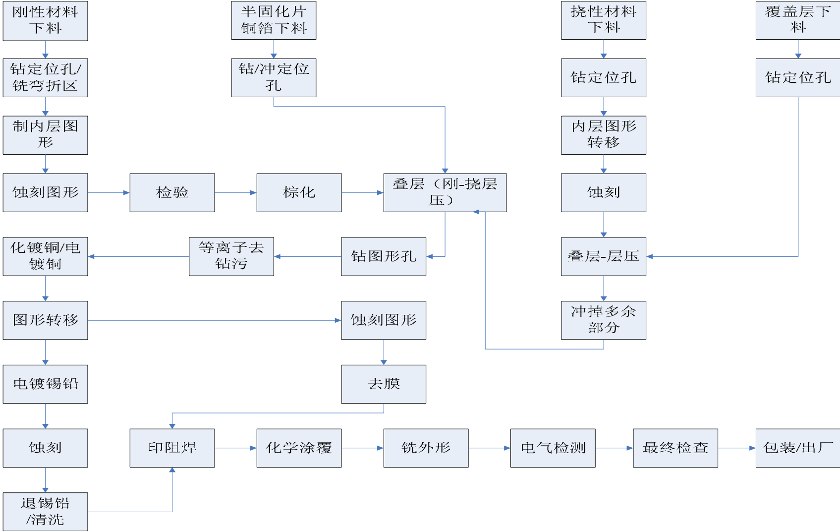
刚挠印制板的工艺流程
