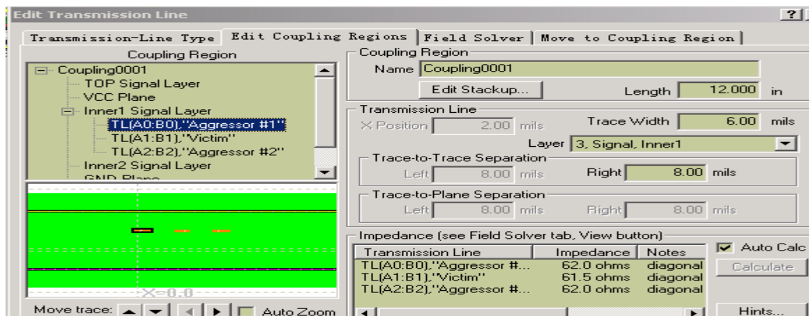
图 3.3 右键点击黄框出现的“Edit Transmission Line”窗口
