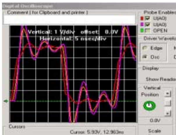
图 1.4 仿真结果
