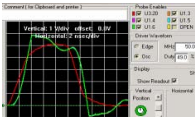
图 5.7 网络 datald 的仿真
