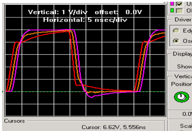
图 1.6 终接负载后的仿真结果
