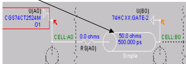
图 1.7 采用 IBIS 数据的电路图
