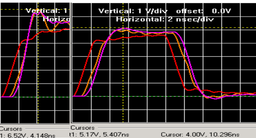
图 4.4 PCB 的 clk 网络仿真（未修正）
