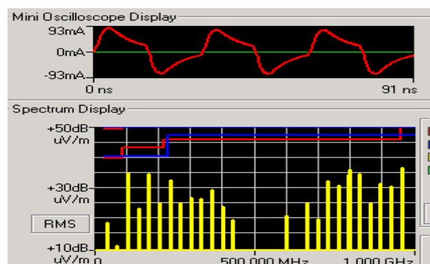
图 2.5 经优化的时钟网络 EMC 仿真
