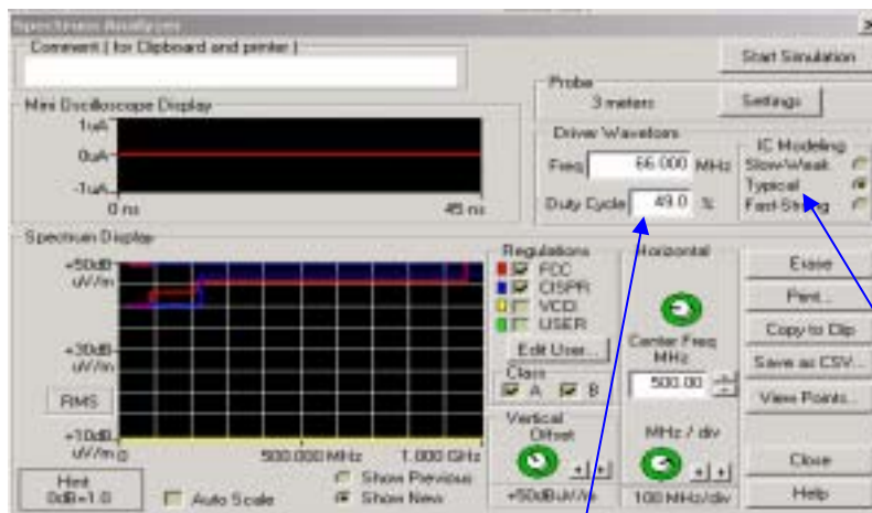
图 2.1 Spectrum Analyzer 窗口
