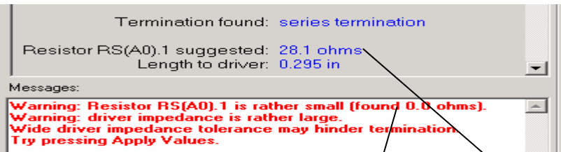
图 1.12 自动优化 原 IBIS 中 0 欧姆 = 》 28.1 欧姆
