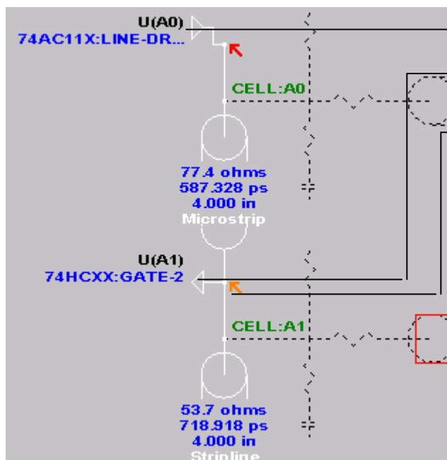
图 1.1 LineSim 图
