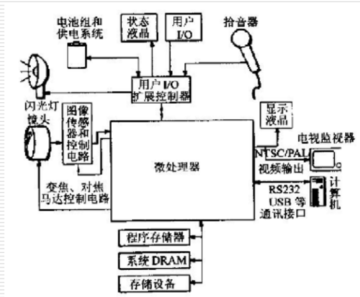
数码相继系统框图
