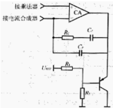
图 5 电流放大器的箝位电路
