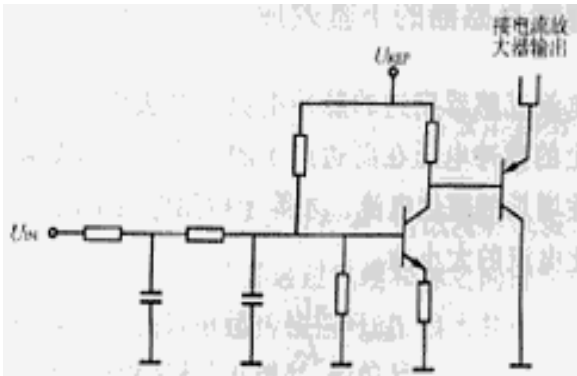
图 6 具有输入电压补偿的电流放大器箝位电路
