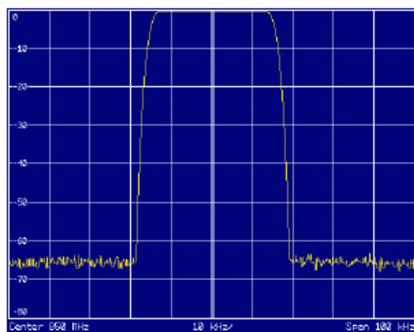
图2-38 在测量IS95邻道功率中30kHz信道滤波器的频率响应
