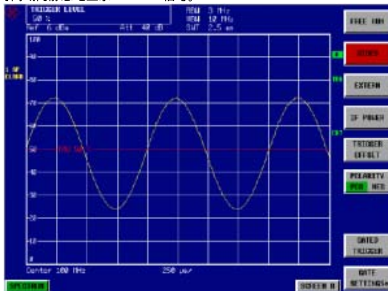
图2-30 由1 kHz调幅载波测量AF信号
