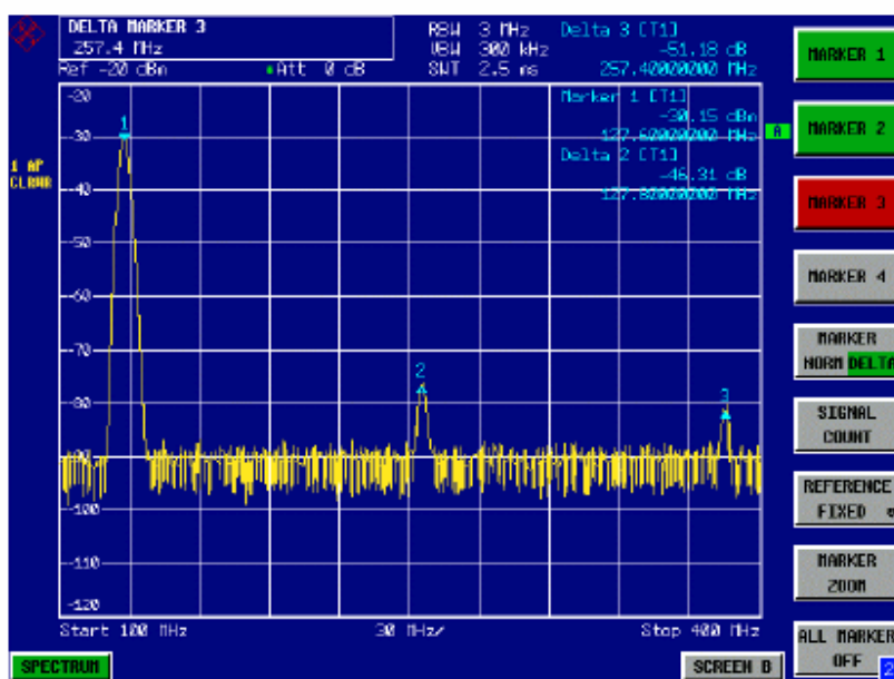
图表.2-3 测量内部基准信号发生器的谐波距离，增量标记2和增量标记3显示了基波和二次谐波、三次谐波之间的距离。
