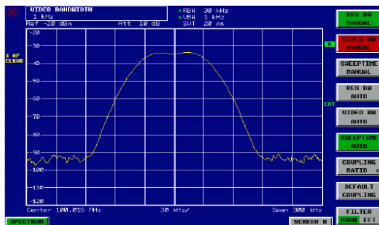
图表.2-9测量两个电平相同的正弦波信号，分辨率带宽根据两个信号的频率差而不同
