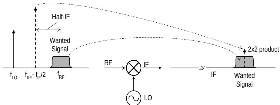
图 3. 半中频干扰
