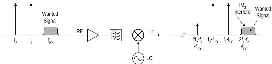
图 4. 双音干扰
