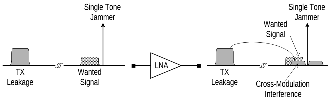
图 2. 交叉调制
