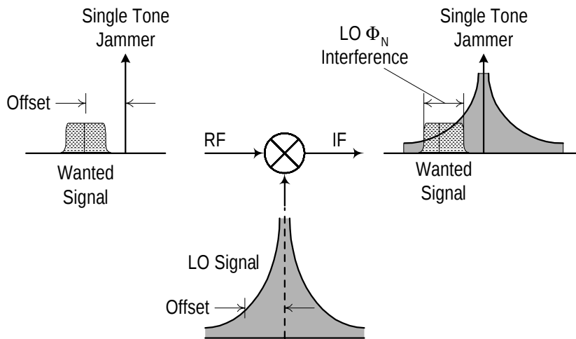
图 1. 互易混频
