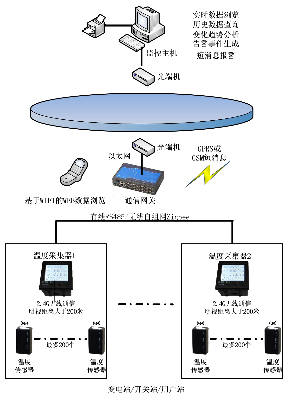
无线温度传感器结构图
