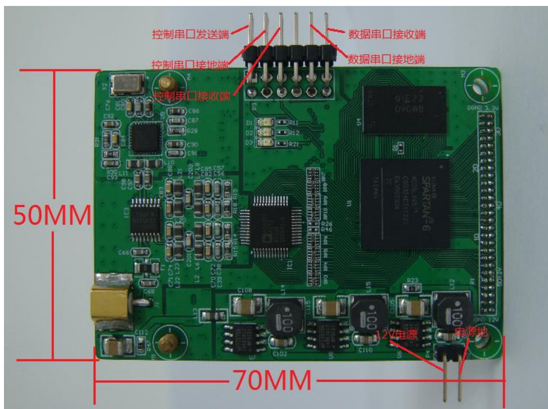
模块上面
