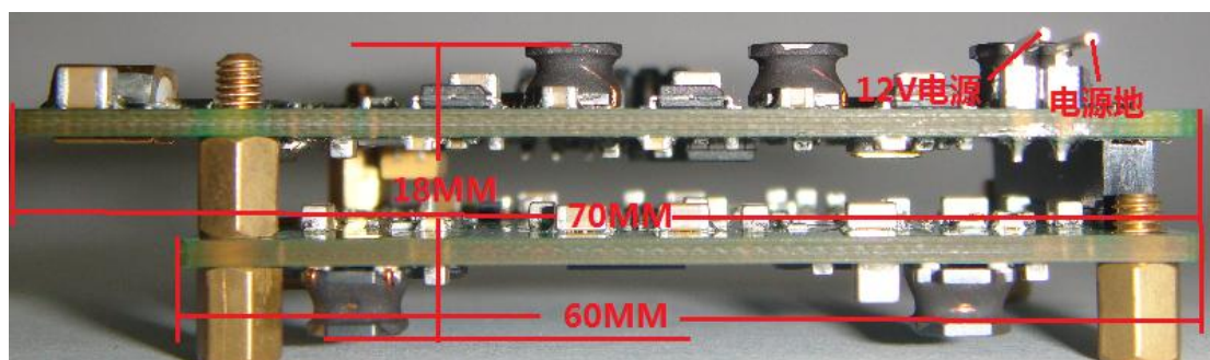
模块侧面
