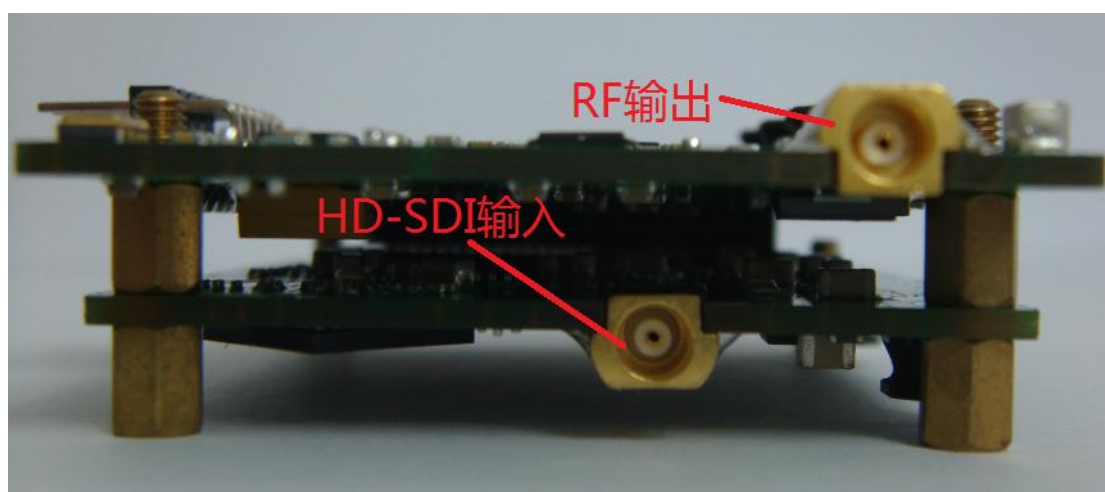
模块前面
