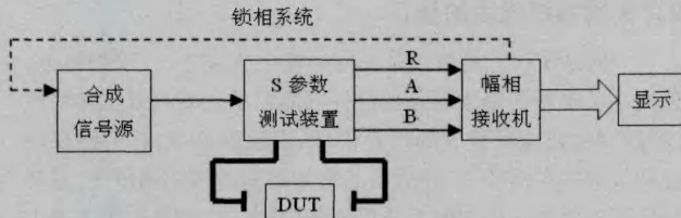
图 1 矢量网络分析仪原理框图
