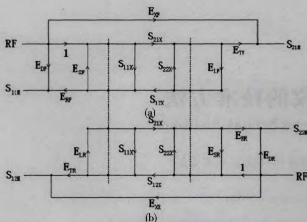
图2 双端口12项误差模型
