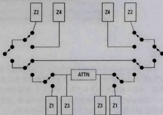
图3 Ecal模块示意图框图
