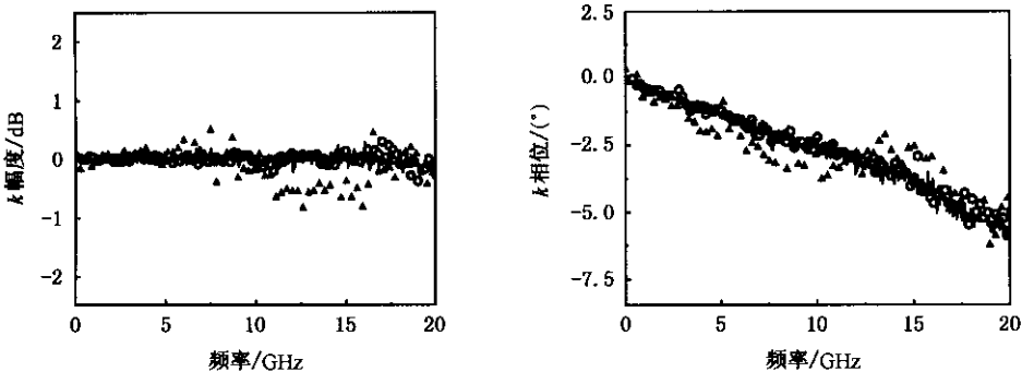
图) 图中实线表示夹具G i 的校准参量 k 的直接测量数据,空心圆和实心三角形分别为本文的校准方法和416校准方法的结果
