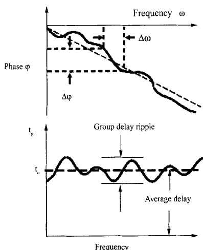
图3 群时延的图像化表示
