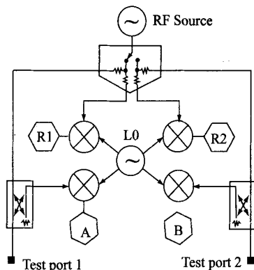
图 1 VNA 网络分析仪的结构图
